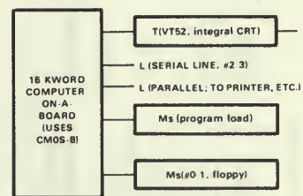
(d) VT78 computer-in-a-terminal.
