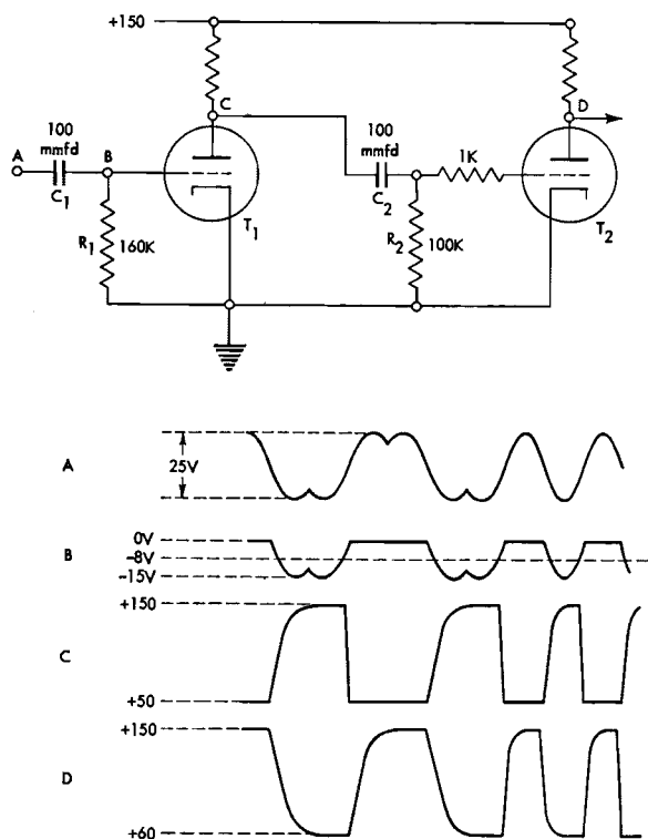
Figure II-25. Shaping Amplifier SA 506
