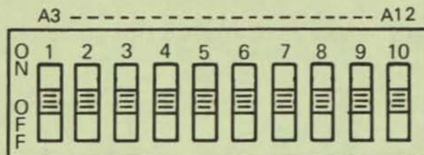
Switch Pack E127
