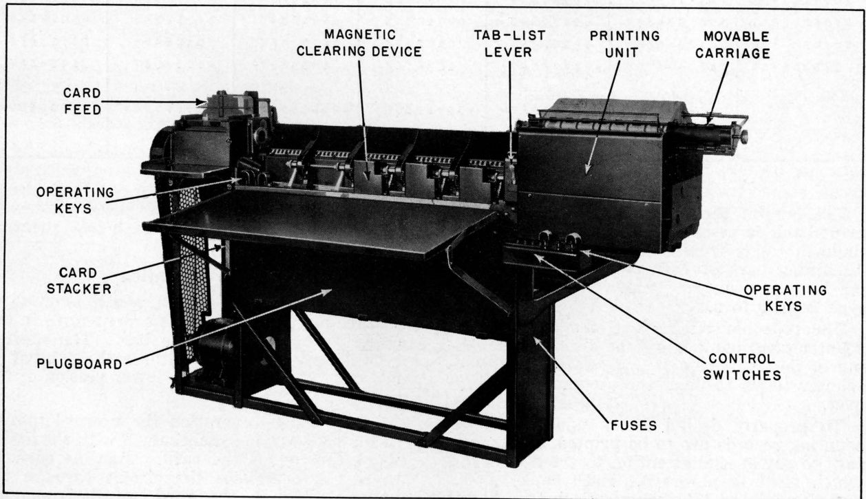
Printing Tabulator
